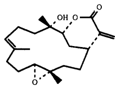
alcyonin
