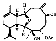
alcyonin
