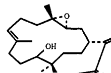
sinulariolide
